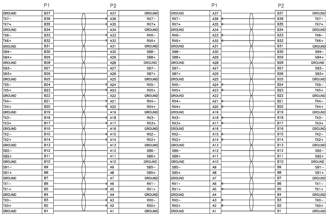
WIRING TABLE
